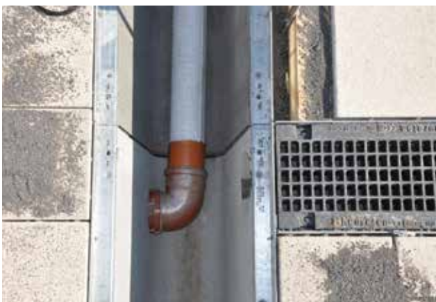
Conexión de los tubos de drenaje al canal DRAINFIX CLEAN.
